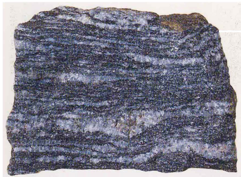
図3 縞状片麻岩帯の泥質片麻岩
